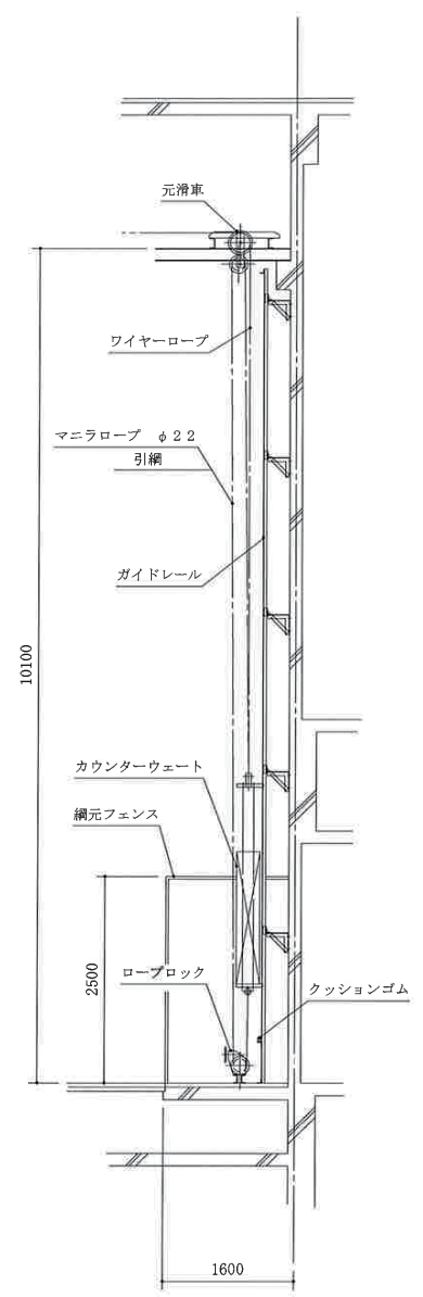
綱元カウンターウェイト部
