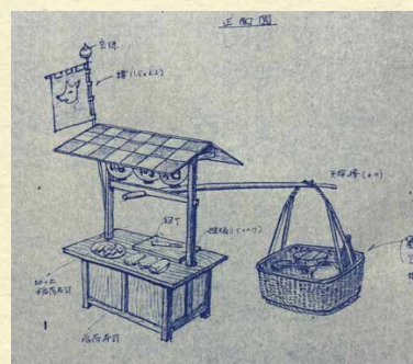
展示実施設計図「稻荷餅屋台」
